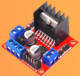
L298N Puente H Módulo 12V
